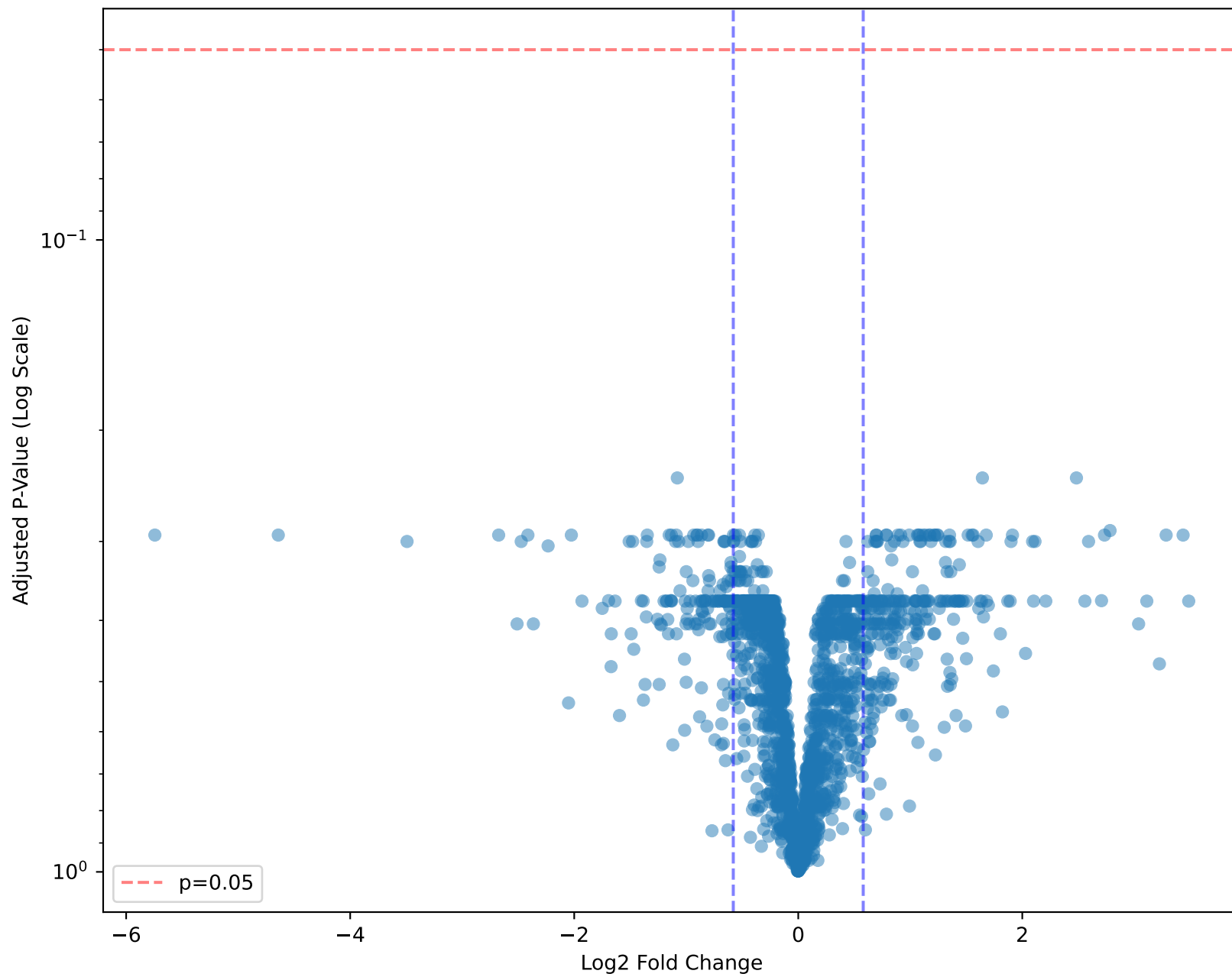
Volcano Plot: D21 - T0
